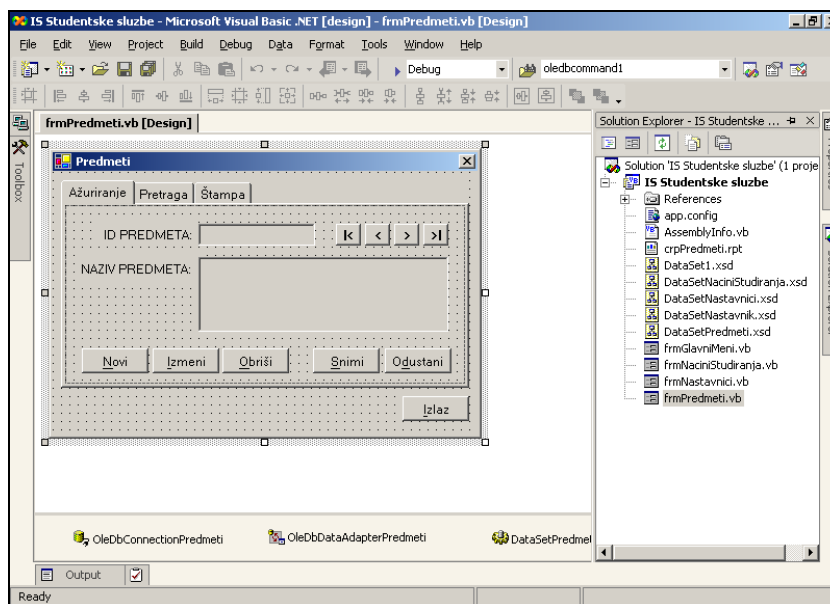
Slika 3.62. Kriiranje kartica na formi
