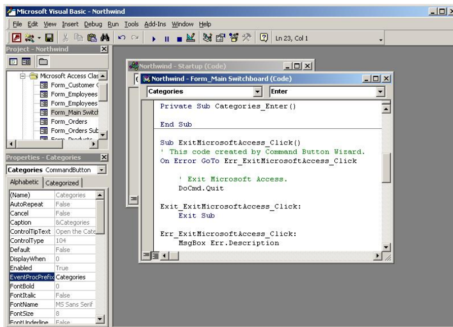
Slika 3.46. Visual Basic Editor
