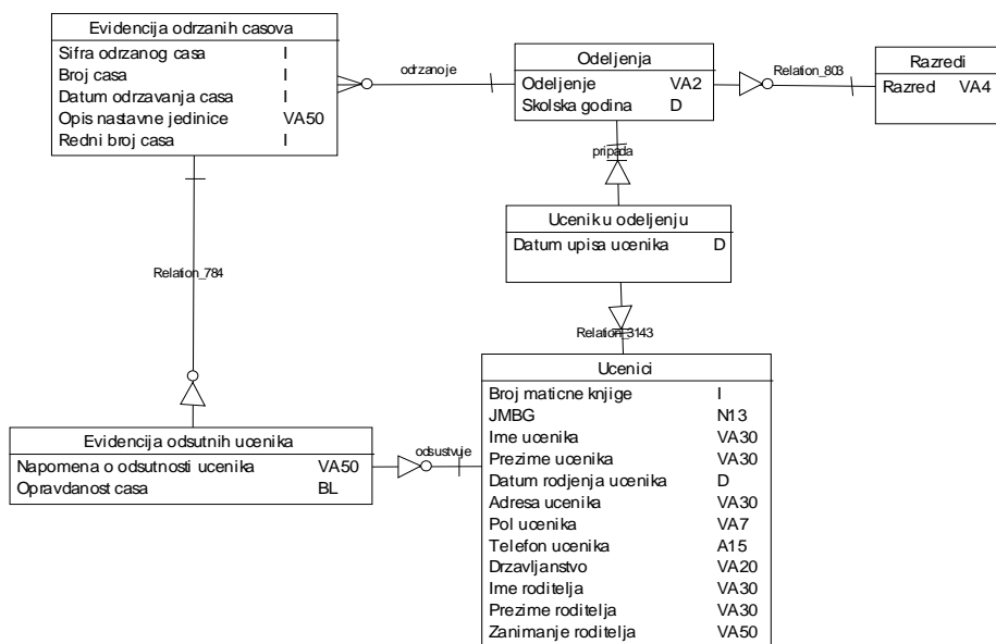
Slika 4.9. Podmodel - Izveštavanje o izostancima učenika za sistem Škola
