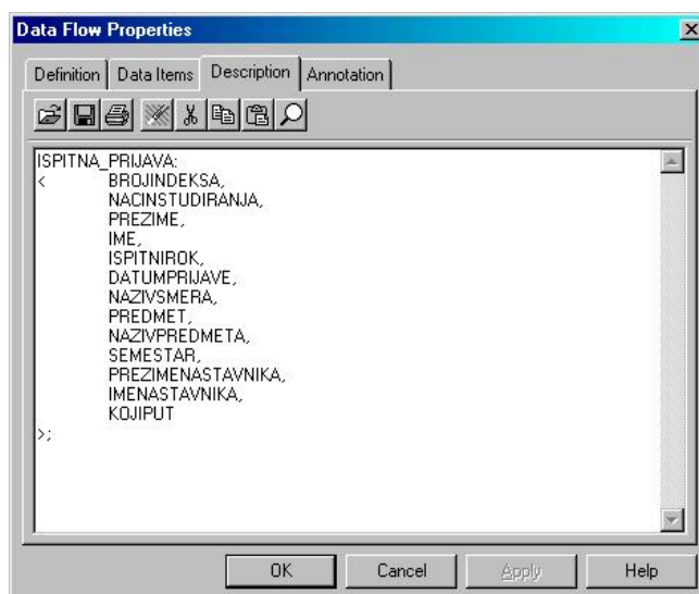
Slika 2.6. Struktura toka podataka
