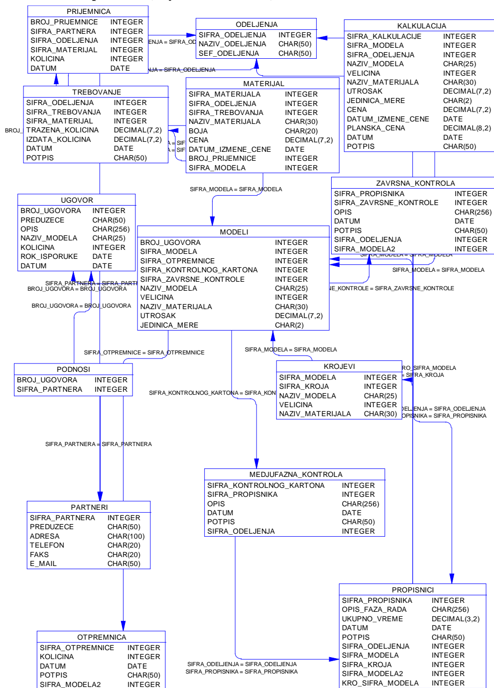
Slika 4.17. Dijagram relacionog modela podataka za sistem Proizvodna organizacija
