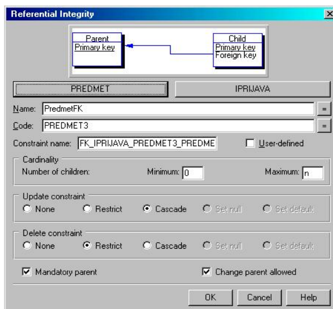
Slika 3.30. Određivanje referencijalnog integriteta
