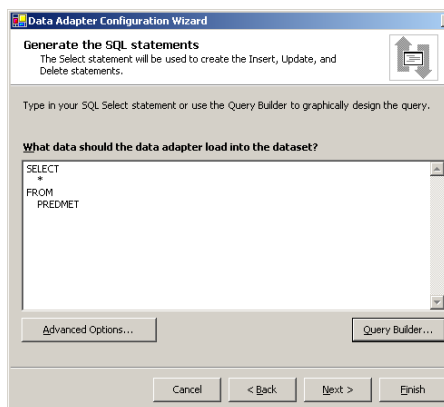
3.65. SQL upit DataAdapter objekta
