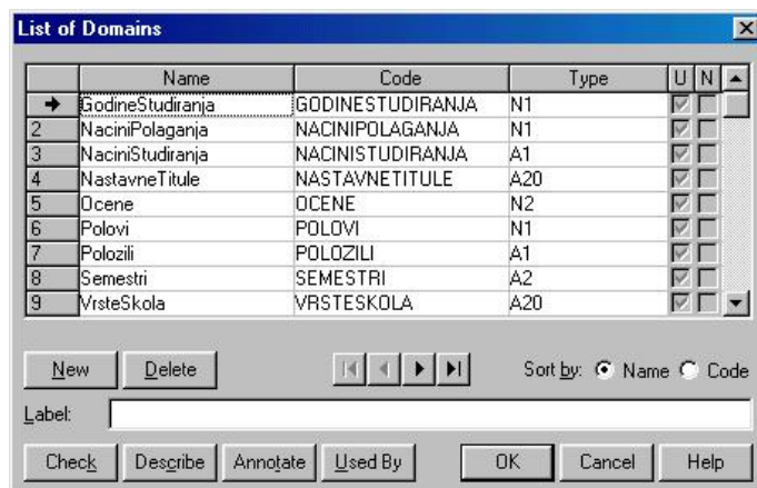
Slika 3.10. Lista definisanih domena
