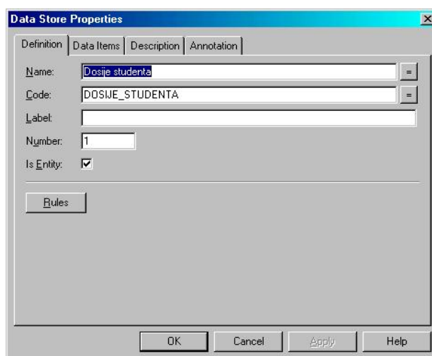
Slika 3.19. Ekran za određivanje osobina entiteta
