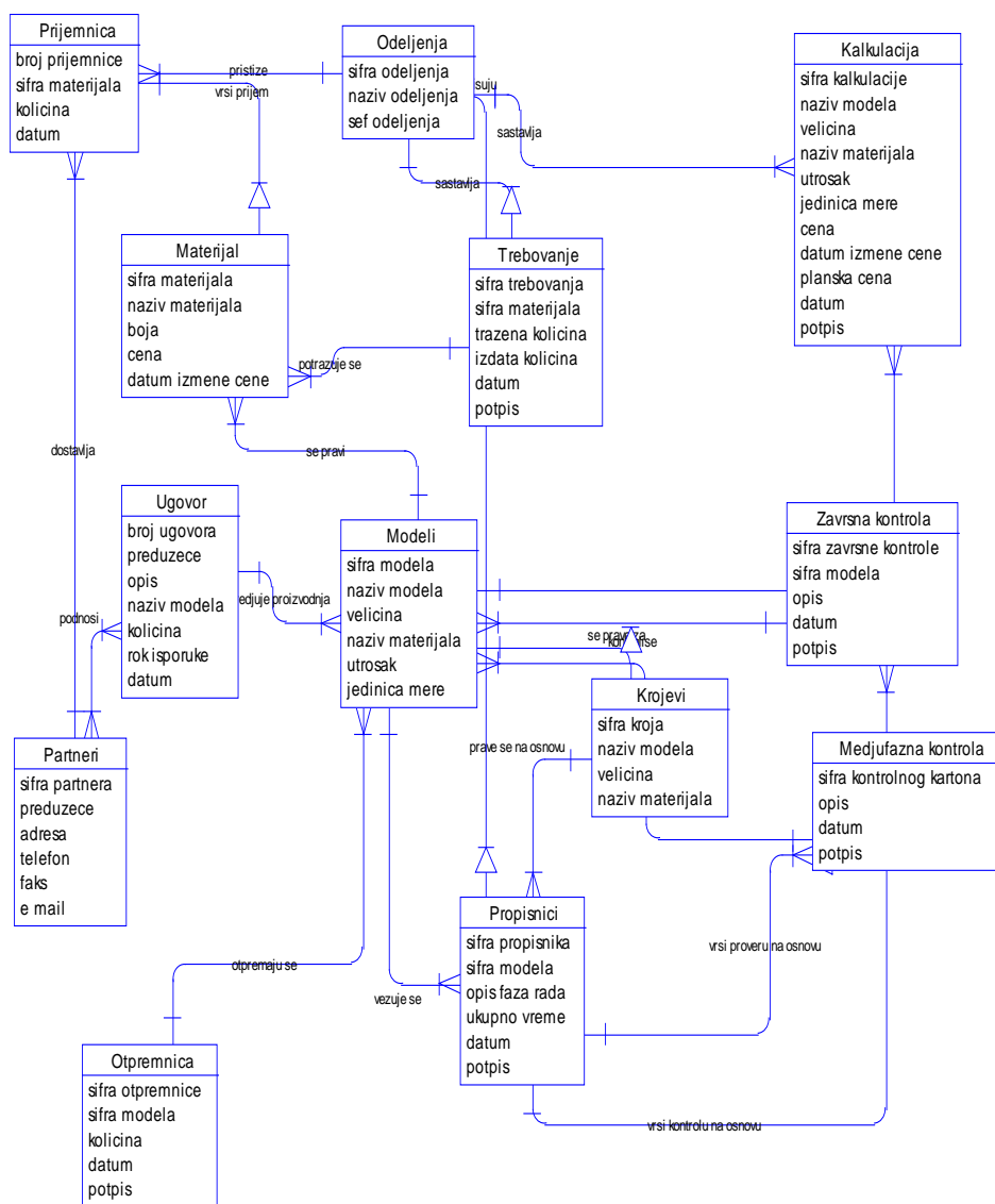
Slika 4.13. Dijagram ER modela podataka za sistem Proizvodna organizacija
