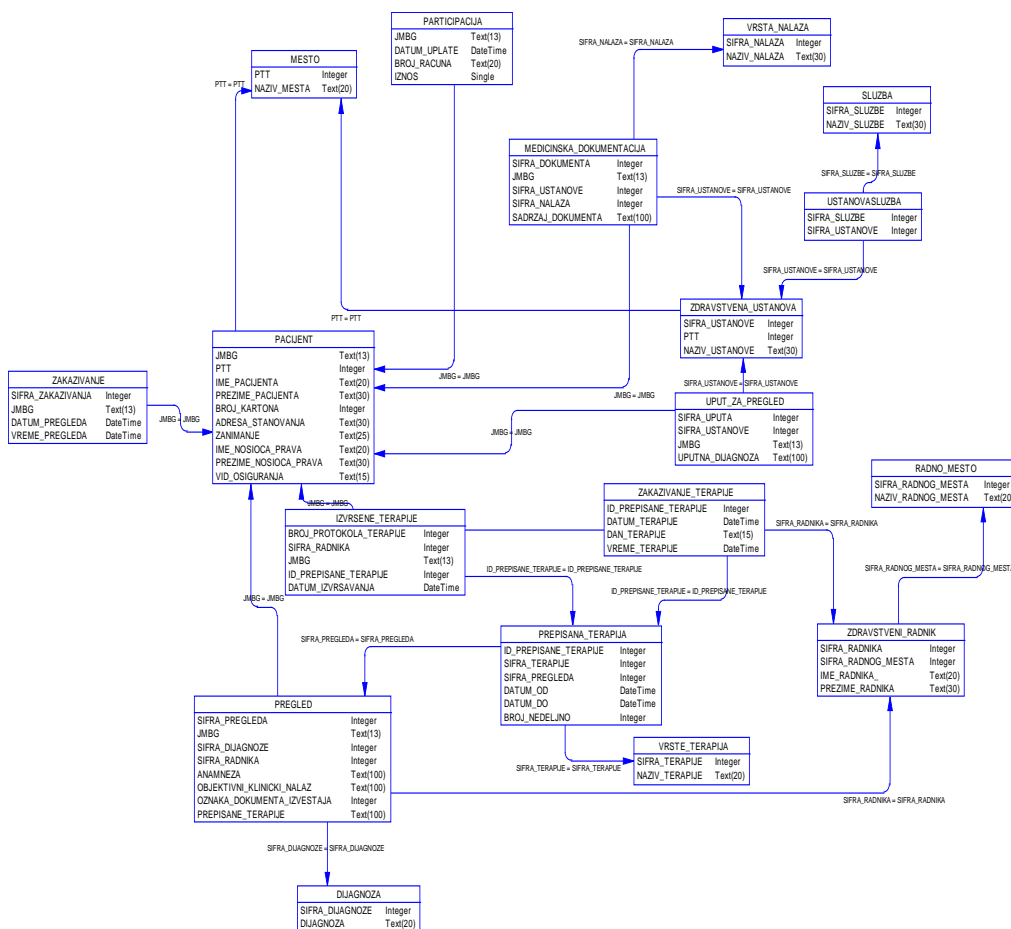
Slika 4.4. Dijagram relacionog modela podataka za sistem Ambulanta
