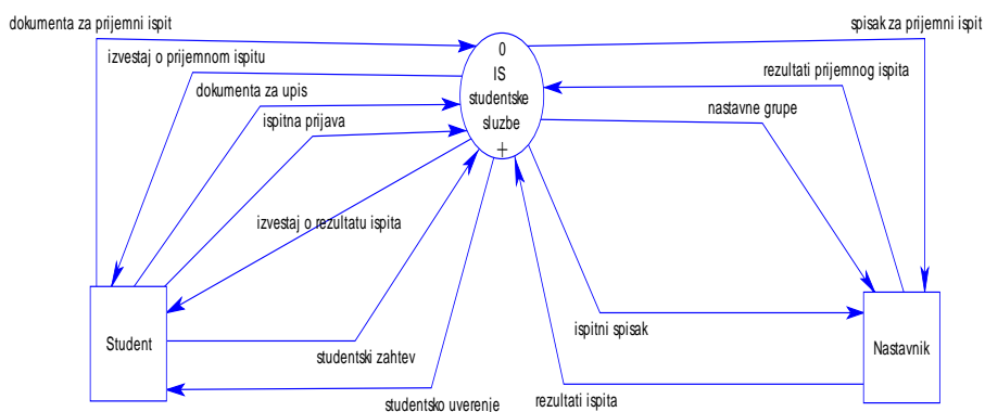
Slika 2.3. Dijagram konteksta SSA
