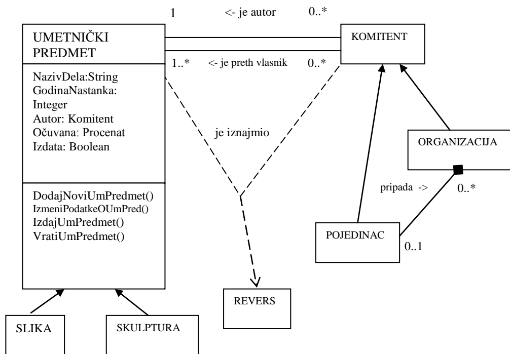
Slika 2.12. CLASS DIAGRAM
