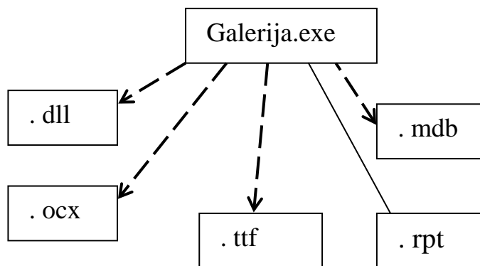
Slika 2.21. COMPONENT DIAGRAM
