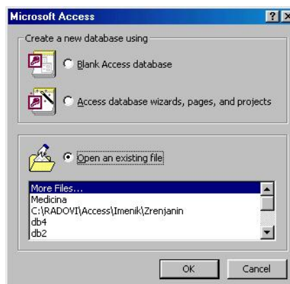
Slika 3.32. Pokretanje Access-a
