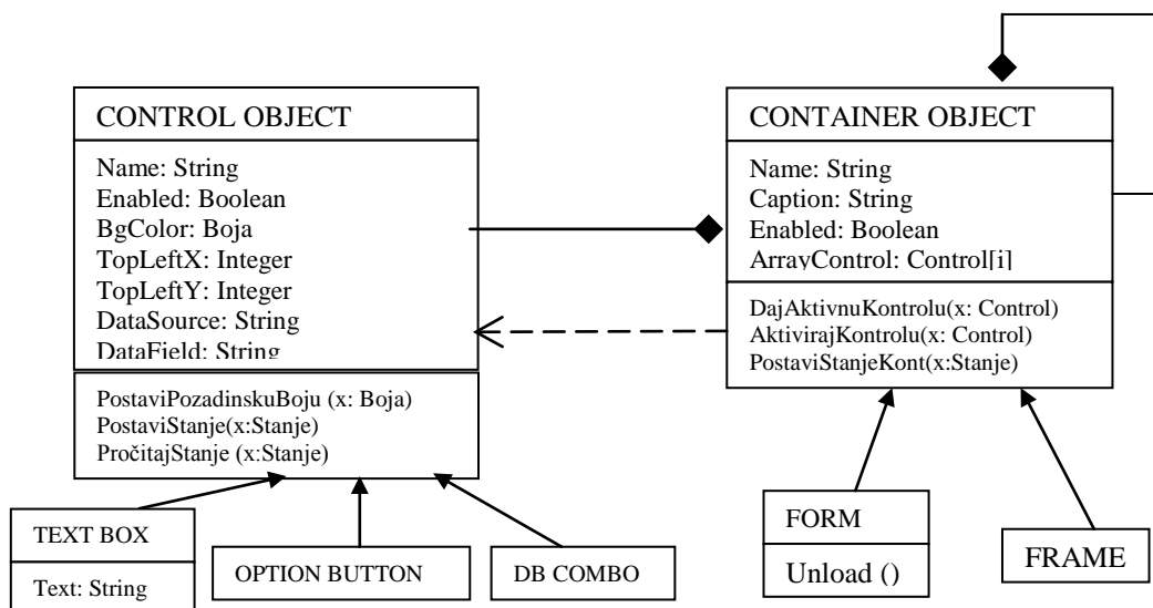
Slika 2.13. CLASS DIAGRAM
