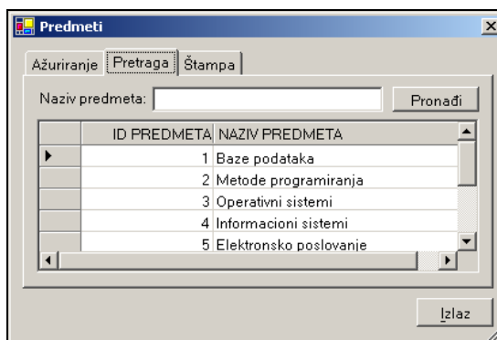
Slika 3.60. Kartica za pretragu podataka na šifarničkoj formi
