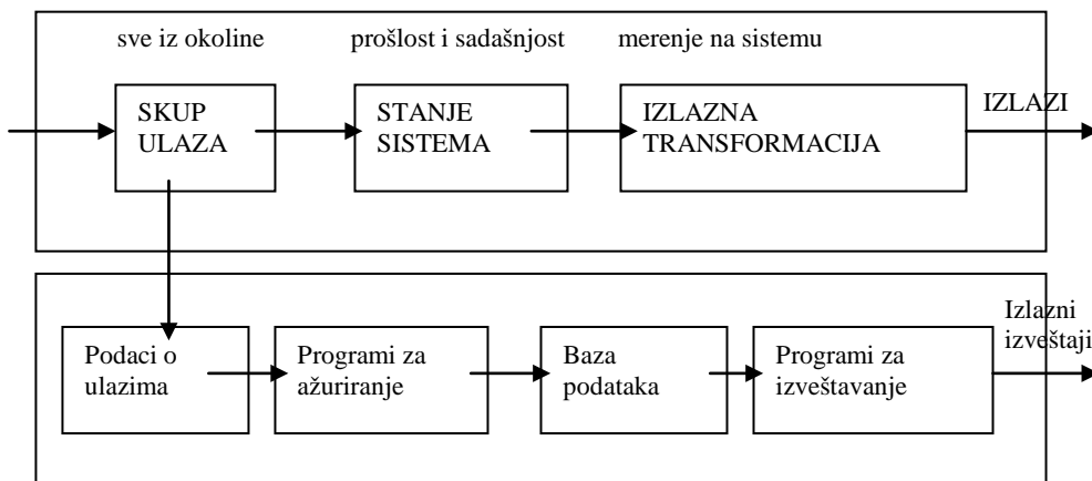
Slika 1.1. Struktura informacionog sistema
