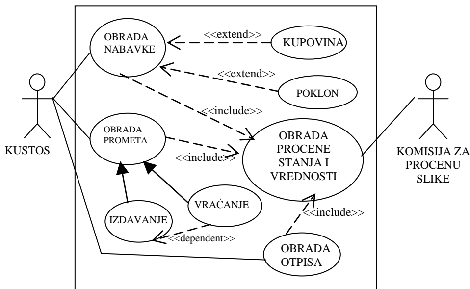
Slika 2.11. USE CASE DIAGRAM
