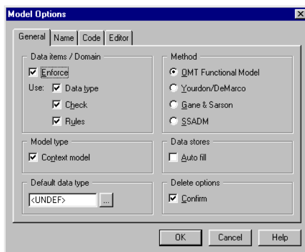
Slika 3.1. Ekran za određivanje vrste modela procesa
