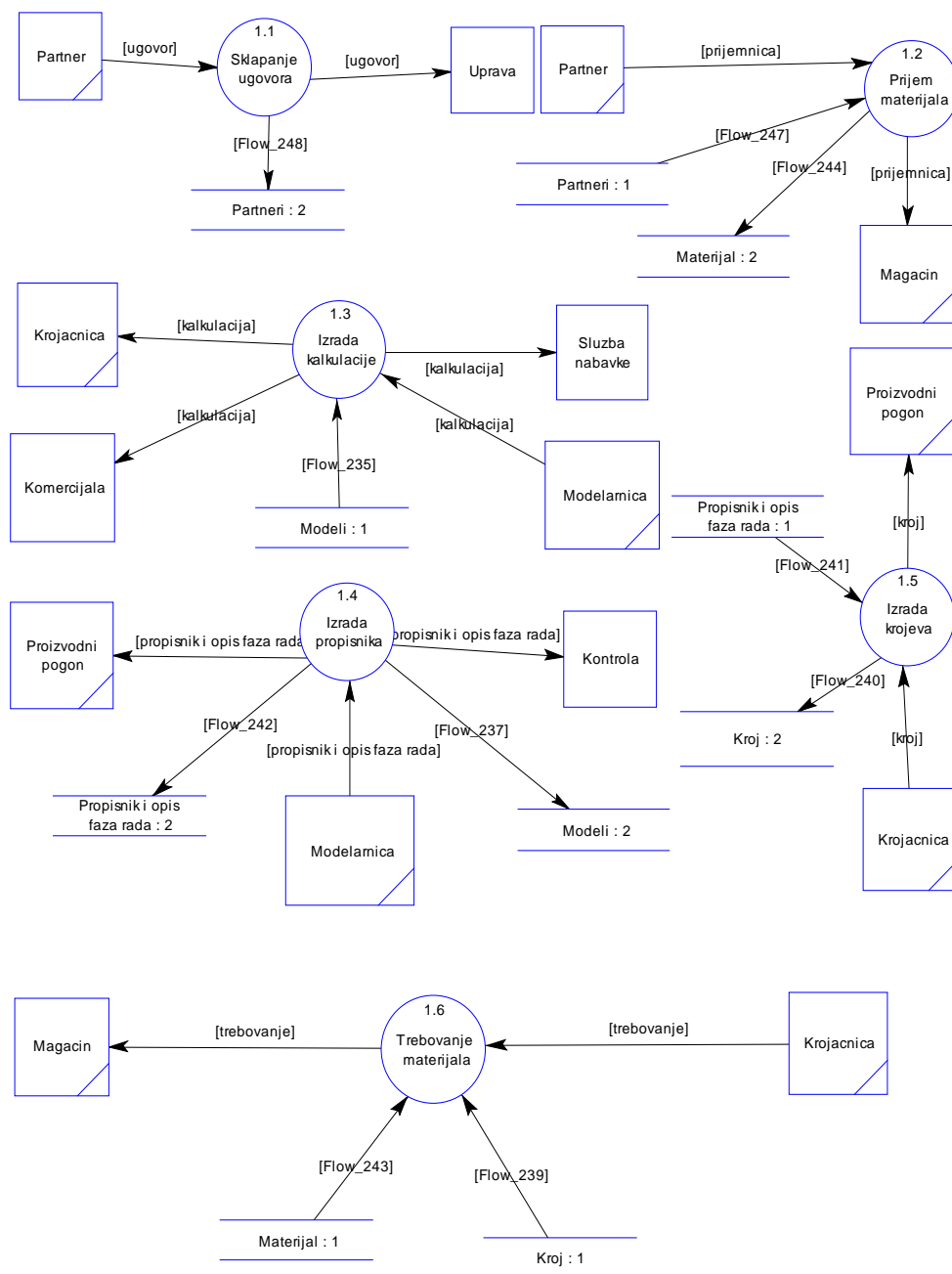
Slika 4.12. DTP 2. nivo za sistem Proizvodna organizacija
