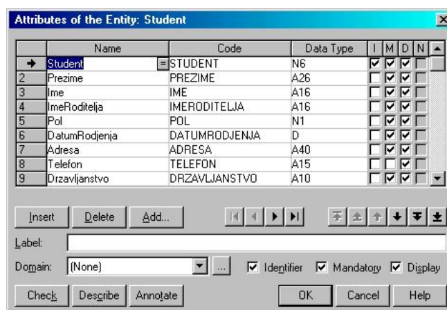
Slika 3.20. Ekran za određivanje osobina atributa
