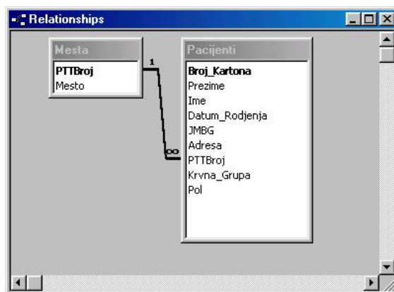
Slika 3.41. Uspostavljena relacija između tabela
