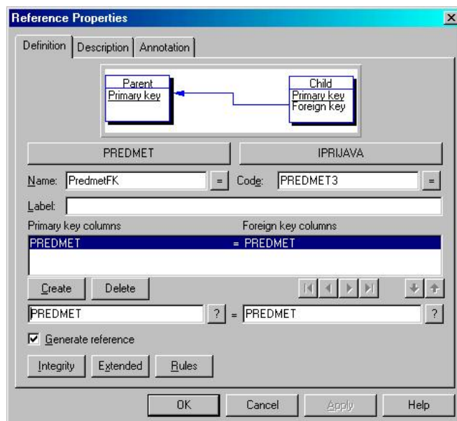
Slika 3.29. Podešavanje osobina relacije
