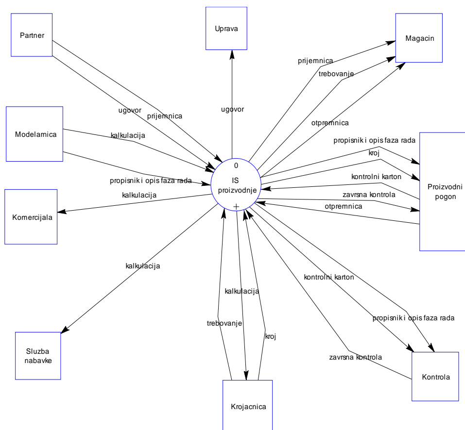
Slika 4.11. Kontekst dijagram za sistem Proizvodna organizacija
