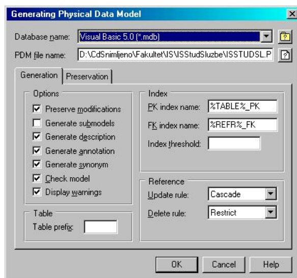
Slika 3.28. Kreiranje fizičkog modela podataka
