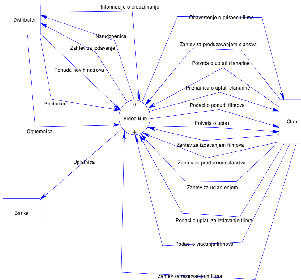
Slika 4.24. Dijagram konteksta za sistem Video klub
