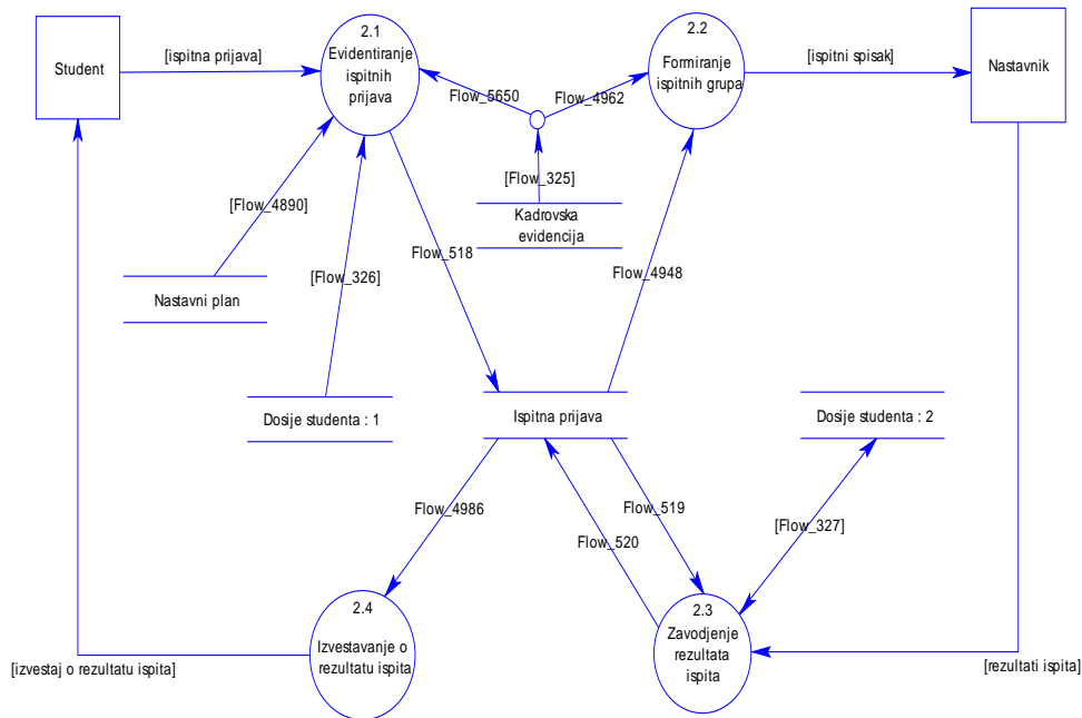
Slika 2.5. Dijagram toka podataka 2. nivo
