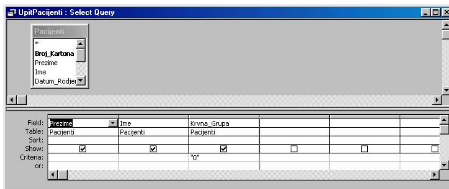
Slika 3.49. Kreiranje upita pomoću QBE
