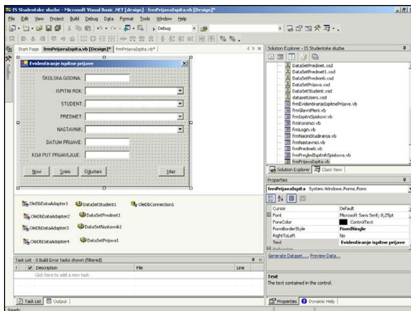
Slika 3.68. Dizajn forme za evidentiranje ispitne prijave
