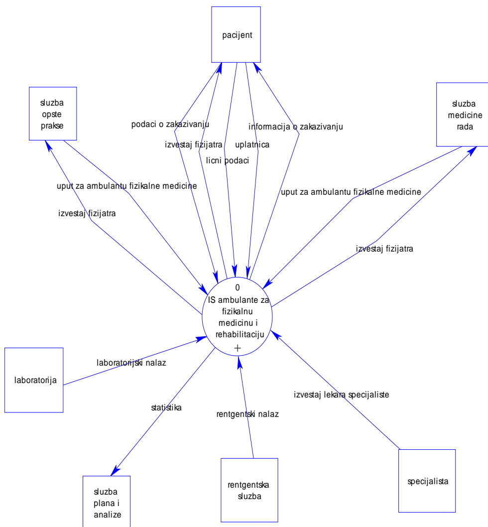
Slika 4.1. Dijagram konteksta za sistem Ambulanta
