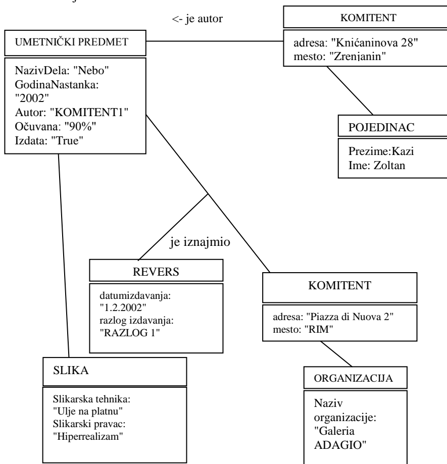
Slika 2.14. OBJECT DIAGRAM
