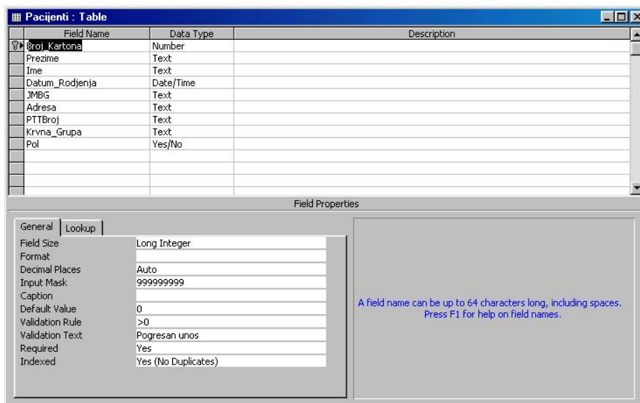
Slika 3.35. Kreiranje tabele
