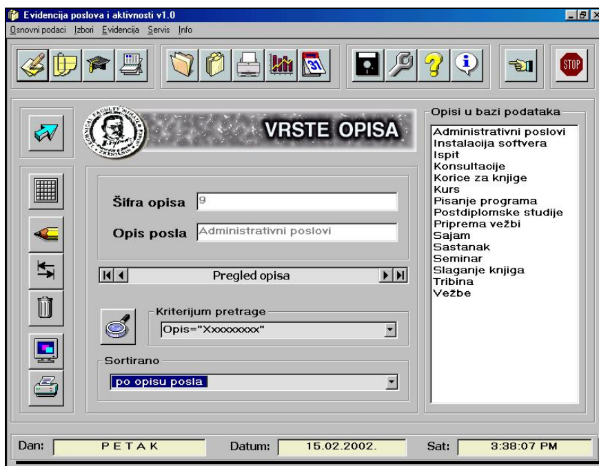
Slika 4.32. MDI forma
