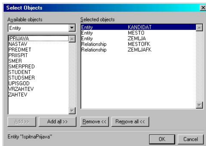
Slika 3.23. Kreiranje podmodela
