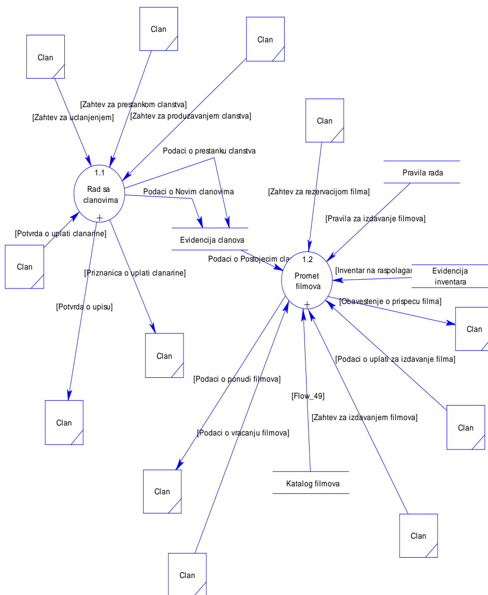
Slika 4.25. DTP 2. nivo za sistem Video klub
