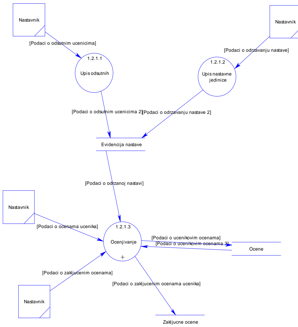
Slika 4.7. DTP 3.nivo za sistem Škola
