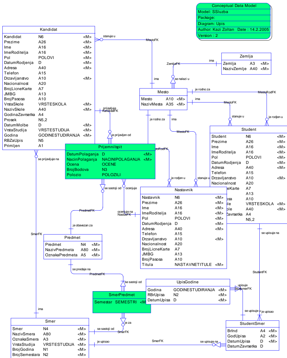
Slika 2.8. ER dijagram u CASE alatu
